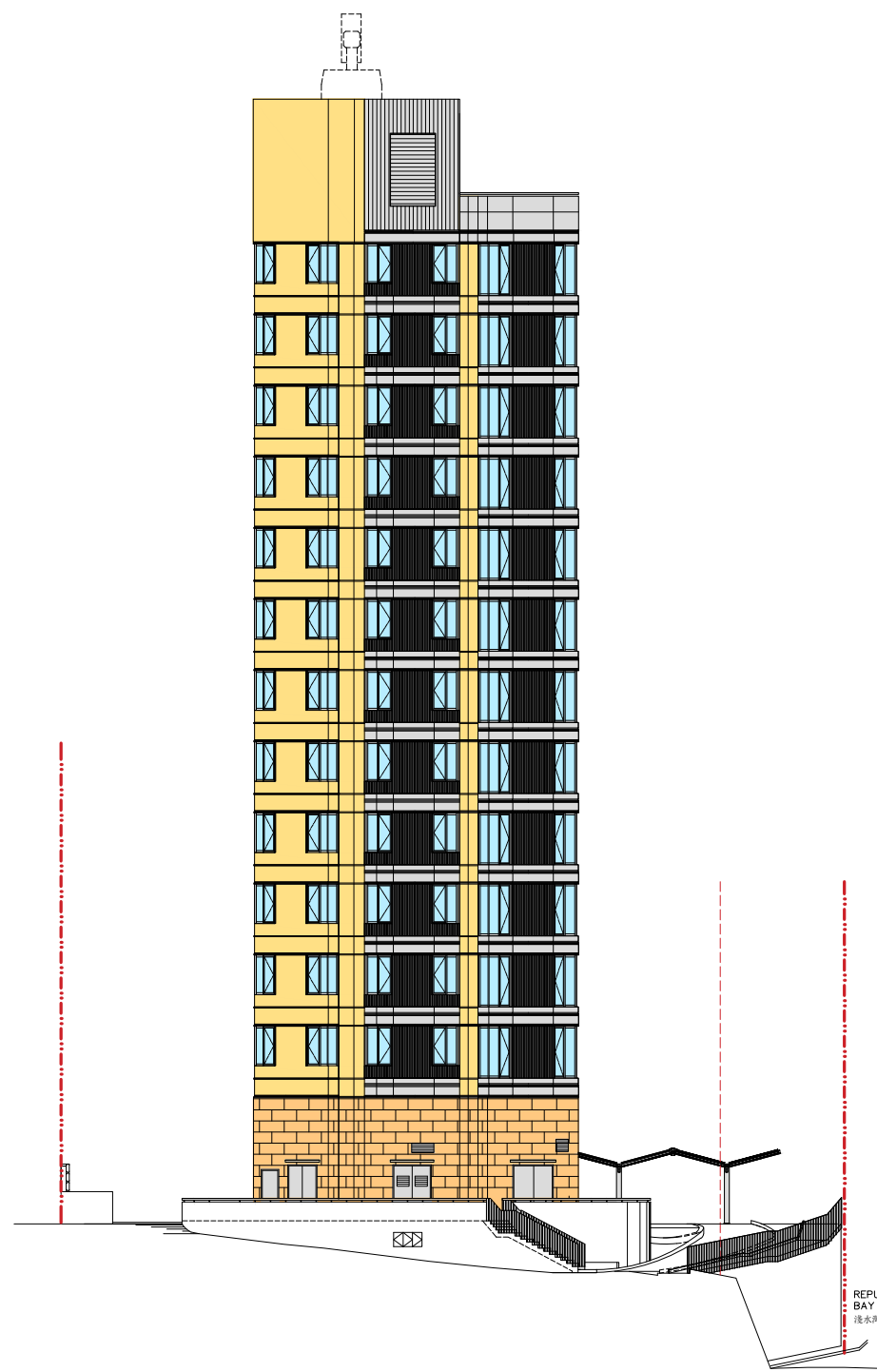
ELEVATION 2 立面圖 2
